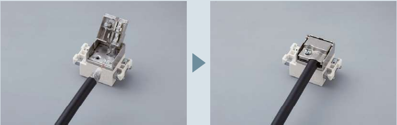
「高シールドらくらく端子」心線を差し込み。 金具をネジ止め(1ヶ所)するだけ。
